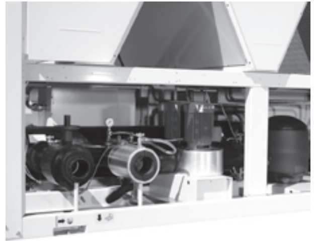
Module hydraulique
